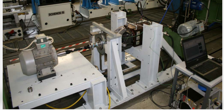
Reibmomentenprüfstand
