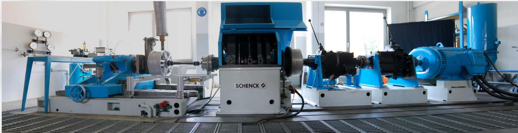
Prüfstand für Triebstrangelemente und Bremsen (110 kW)
