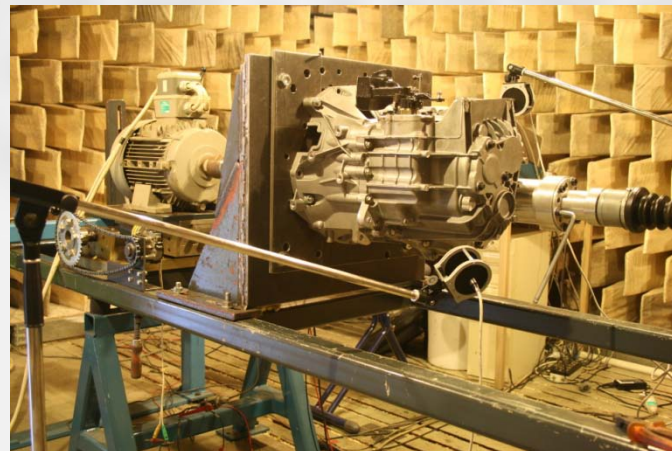
Kleines Schallmesshaus (Halbfreifeldraum) für Komponenten- untersuchungen
